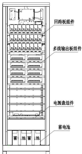
图 2-6 柜式内部结构与连接
