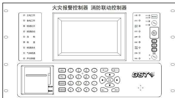
图 2-3 主控面板
