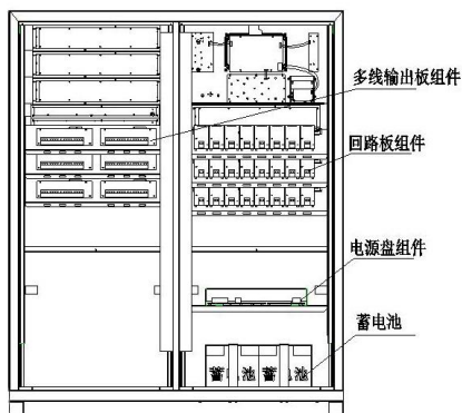
图 2-7 内部结构与连接
